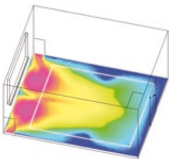
Quelllüftung, feste Außenverschattung
