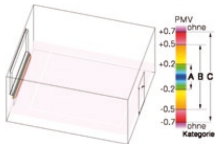
Mittlere Klimabewertung PMV
