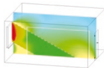
Ohne Verschattung, Fensterflächenanteil 30 Prozent
