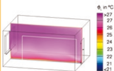
Fensterflächenanteil 30 Prozent, ohne Verschattung
