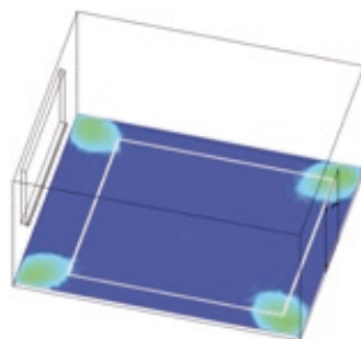
Kühlfußboden, feste Außenverschattung
